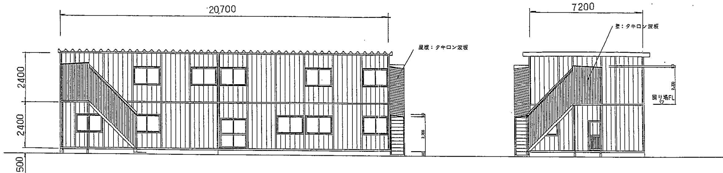
A通立面図 S=1/100
